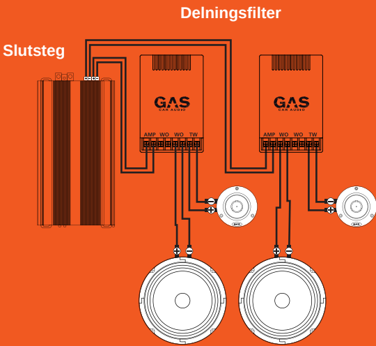
Inkoppling av två midbasar / två diskanter
