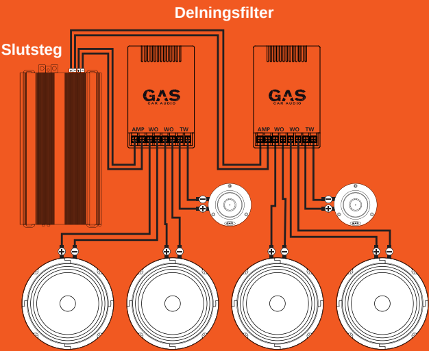
Inkoppling av fyra midbasar / två diskanter
